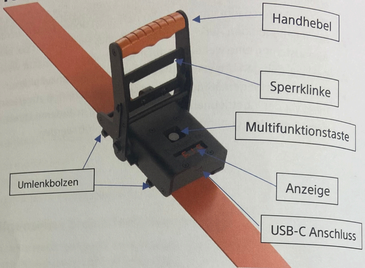
Abb. 1: Bedien- und Anzeigeelemente des DoMessPro
