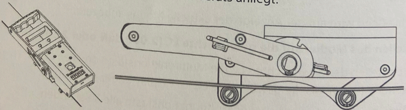
Abb. 2: Korrekte Ausrichtung auf dem Gurtband
